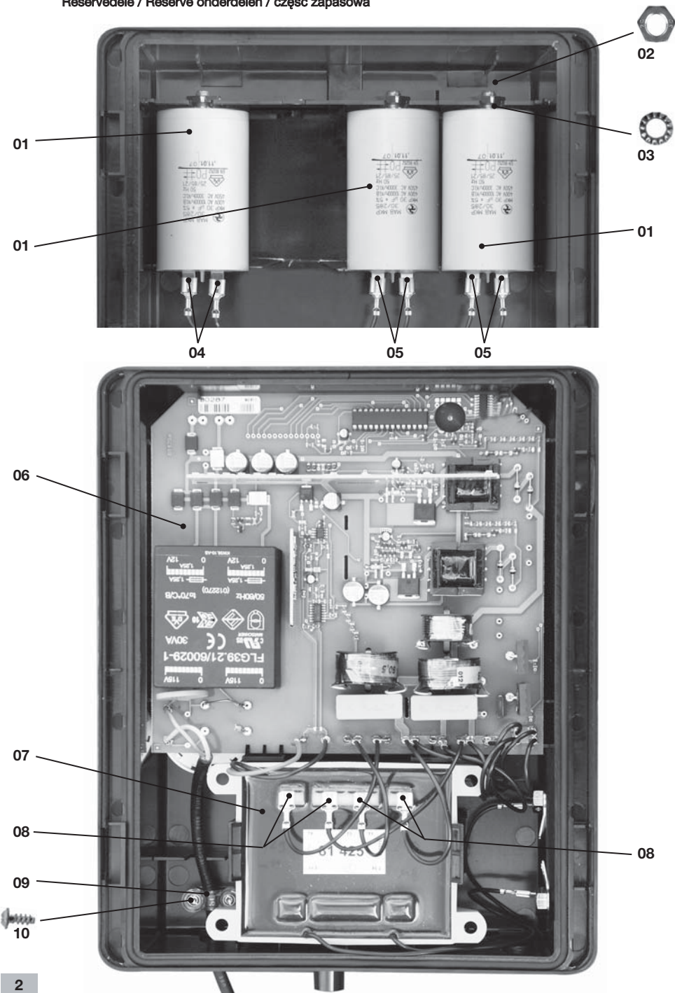
Fig. 1 Ersatzteile / Spare parts / Pièces détachées / Peças / Pezzi di ricambio / Reservedele / Reserve onderdelen / część zapasowa
