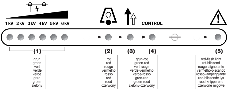
Fig. 3 / LED-Test
